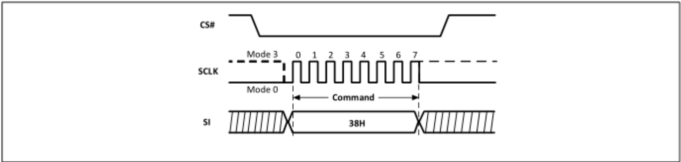
Figure-75. Enable QPI (QPI)
